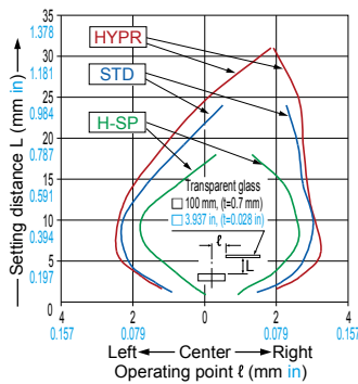
FD-L30A
