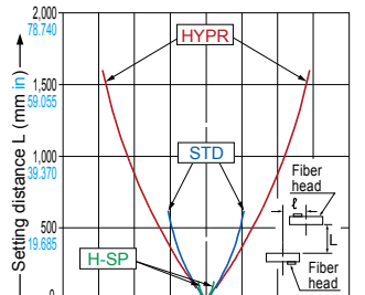
FT-Z20W
