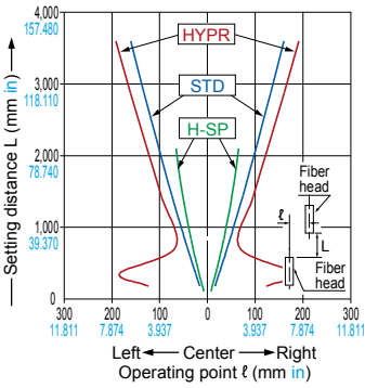
FT-AL05
